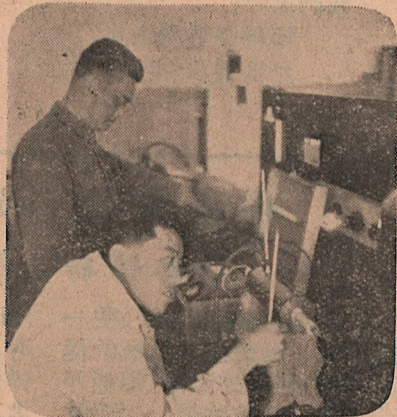
該組主任和教师在傳热實驗室研究實驗中的問題。(鋼士攝)
